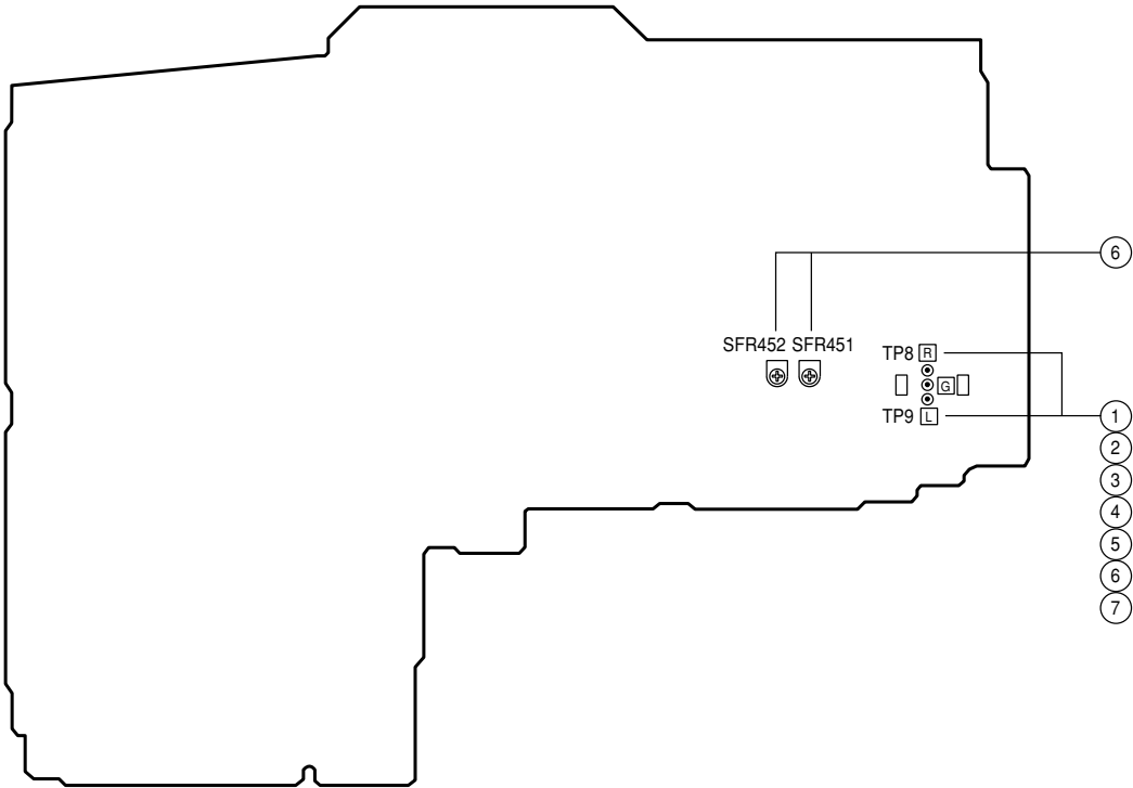
MAIN C.B (PATTERN SIDE)
