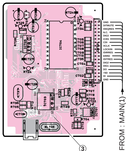
P.C.B DIGITAL
